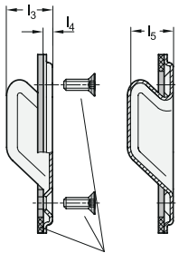
Wkręty uszczelniające z tłem stożkowym / uszczelka kasety (nr. identyfikacyjny 2)
